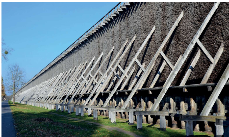
Tężnie w Ciechocinku są największa tego typu budowla w Europie
