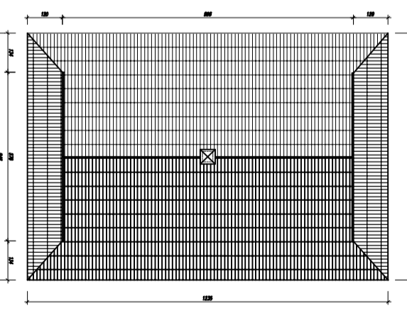
PROJEKT BUDOWLANY DESZCZOCHRONU SKALA 1:50
