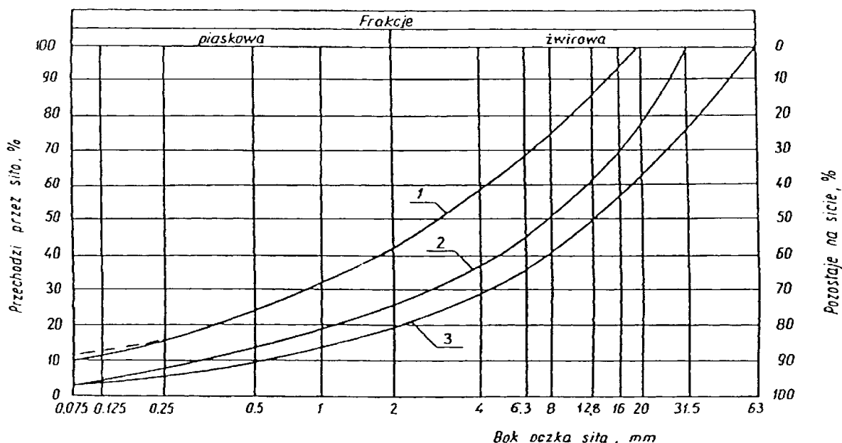
Rysunek 1. Pole dobrego uziarnienia kruszyw przeznaczonych na podbudow wykonywane metodą stabilizacji mechanicznej
